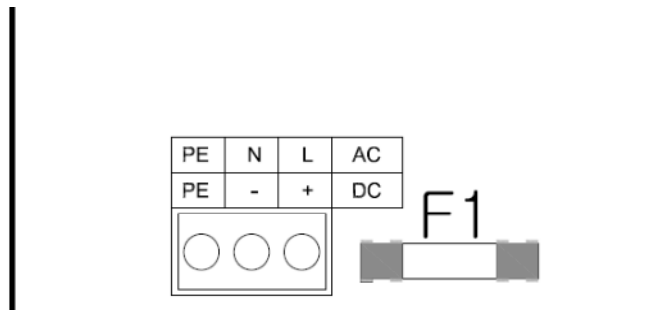
Afbeelding 4 Aansluiting netstroomkabel
