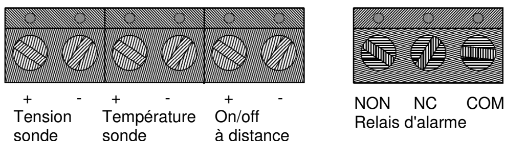
Illustration 3 Bloc connecteur
